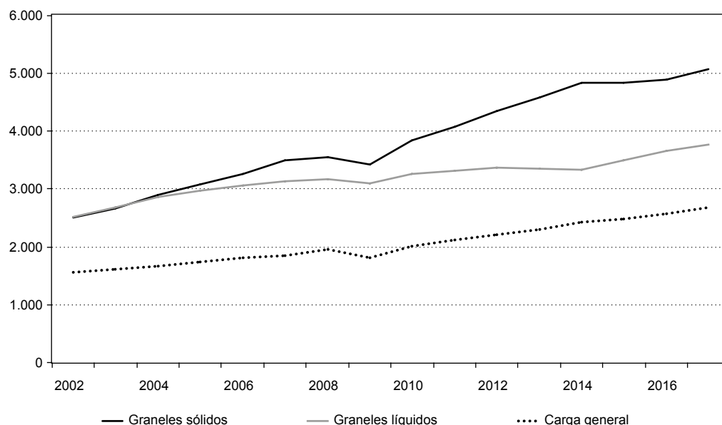
GRÁFICO 1 EVOLUCIÓN DEMANDA DE TRANSPORTE MARÍTIMO POR GRUPOS DE PRODUCTOS (En millones de toneladas)
